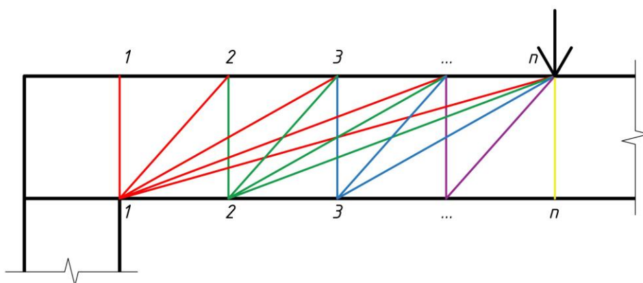
Рисунок 16.12. Назначение расчетных наклонных сечений
