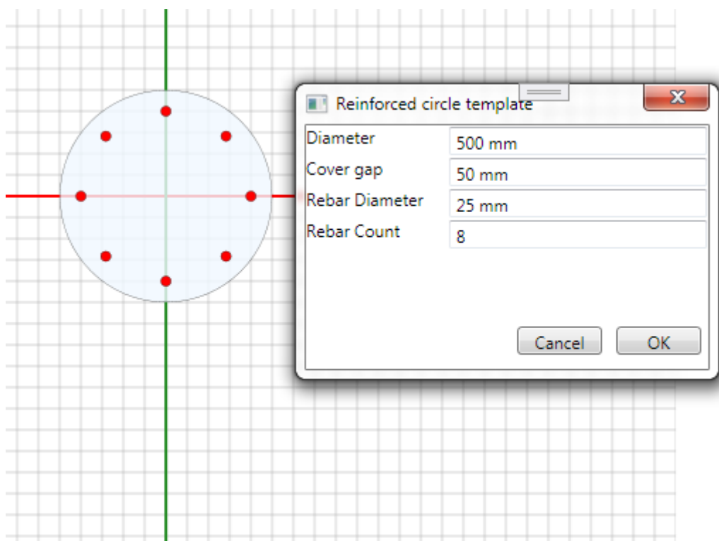
Рисунок 10.3. Шаблон круглого сечения железобетонного элемента. В настоящий момент вы можете использовать следующие виды шаблонов:
